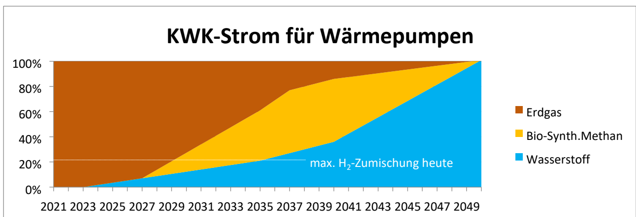
Abbildung 2: Energieformen für die KWK-Anlagen für Heizungen für Haushalte und GHD
