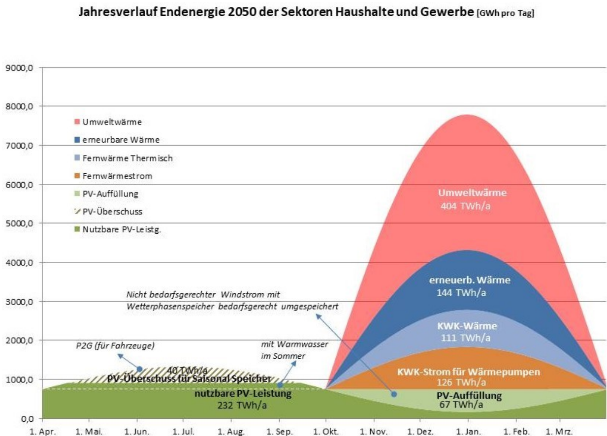
Abbildung 1: Jahresverlauf und Zuordnung des Energiebedarfs von Haushalten und GHD
